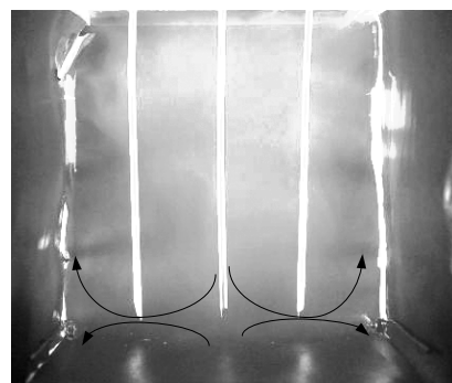
รูปที่ 4 - 10 ภาพลมหมุนวนในระนาบหน้าตัดท่อทดสอบเมื่อ H = -3.75 cm, G = -3.75 cm
