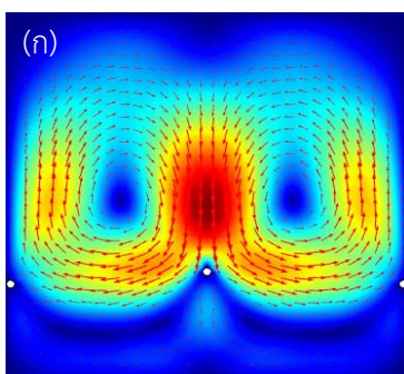
รูปที่ 4 - 7 ภาพลมหมุนวนในระนาบหน้าตัดท่อทดสอบที่จำนวนแท่งอิเล็กโทรดค่า n ต่างๆ (ก) 1 แท่ง (ข) 2 แท่ง และ (ค) 3 แท่ง
