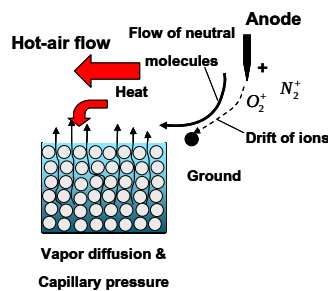
รูปที่ 2 กลไกการเกิดลมหมุนวนในทิศการไหลของลมเพื่อการถ่ายมวลและความร้อนในแพคเบตโดยใช้สนามไฟฟ้า [5]
